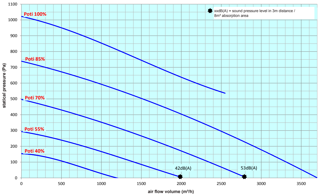
pst-V - diagram
