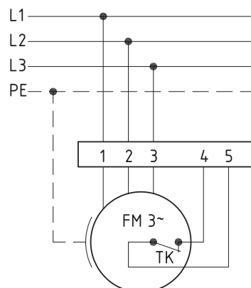
Anschlußplan 0.13-2 I.
