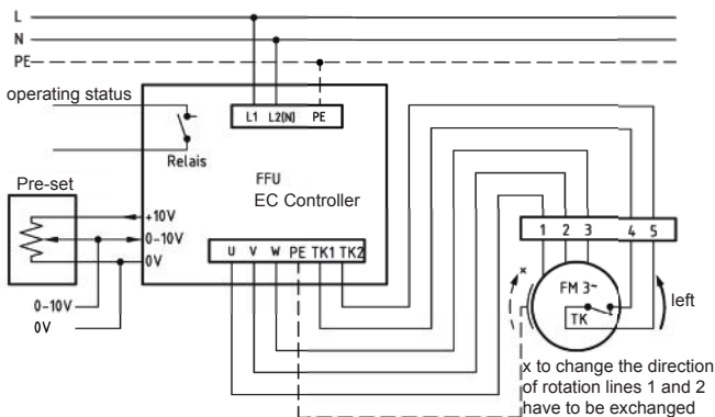
FFU-EC 230
