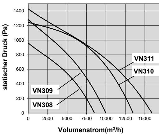
Größe 3 - 1000x1000x850 mm
