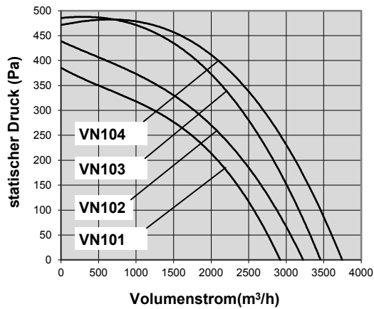
Größe 1 - 600x600x600 mm
