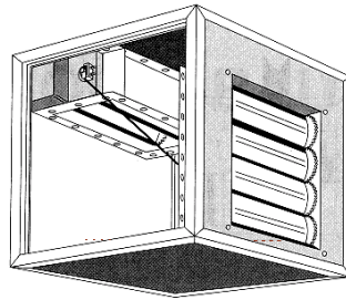
Normbaureihe LM ...
