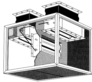
Normbaureihe CLM ...
