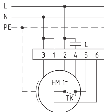
Anschlußplan 0.11-1 l.
