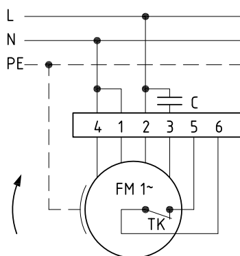
Anschlußplan 0.11-1 r.
