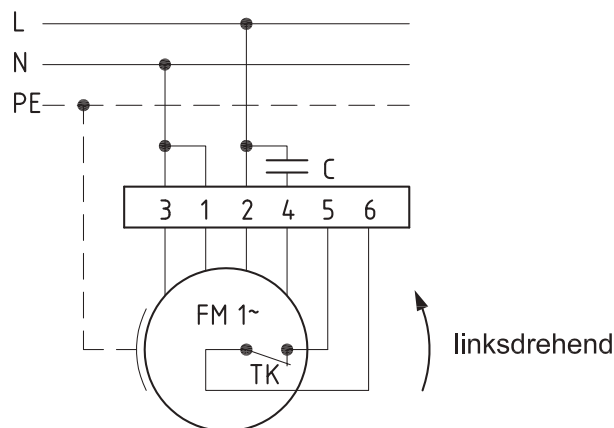
Anschlußplan 0.11-1 I.
