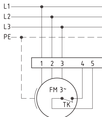
Anschlußplan 0.13-2 I.
