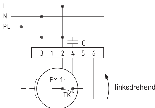
Anschlußplan 0.11-1 I.
