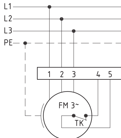
Anschlußplan 0.13-2 I.
